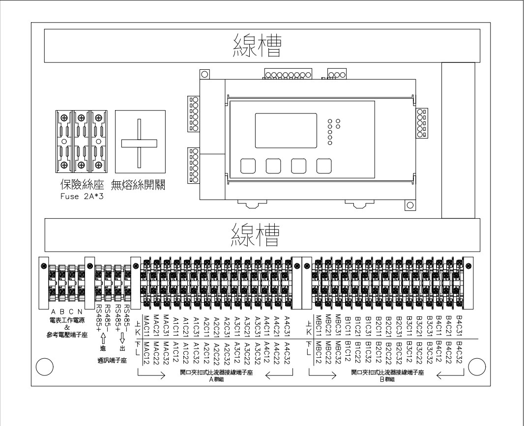
箱體內部
