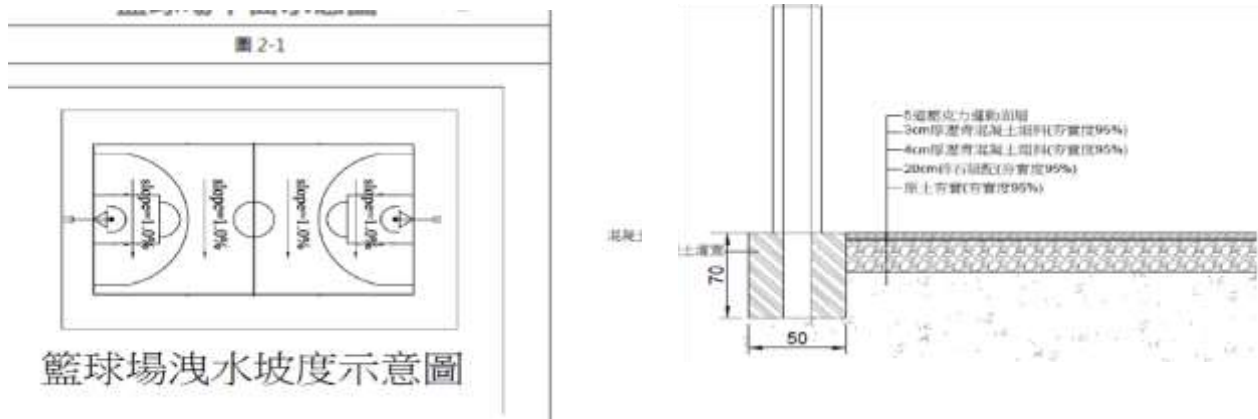
圖 6-1、洩水坡度及面層設計規劃示意圖
